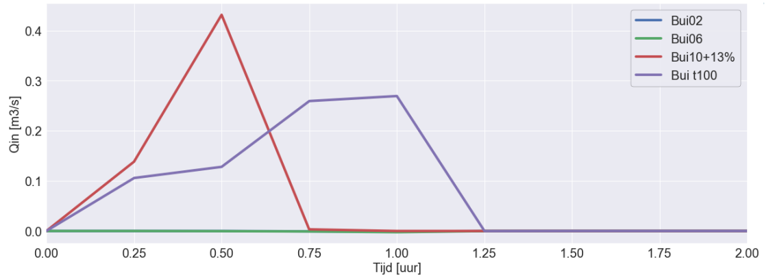
Figuur 4-8: Verloop van ingaande debiet in de wadi voor vier verschillende buien (Bui02, Bui06, Bui10+13% en klimaatbui T100) – ingezoomd op eerste 2 uur van de bui. Het ingaande debiet is ter plekke van de stuwput ten westen van de wadi.
