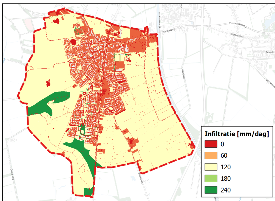
Figuur B5: Infiltratieraster van het integrale model Vries Zuid – huidige situatie
