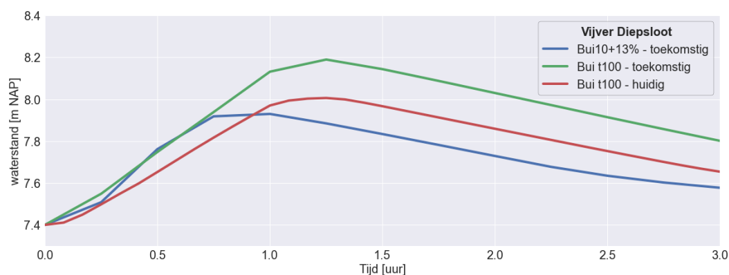
Figuur 4-13: Verloop van de waterstand in de vijver bij Diepsloot voor drie scenario's
