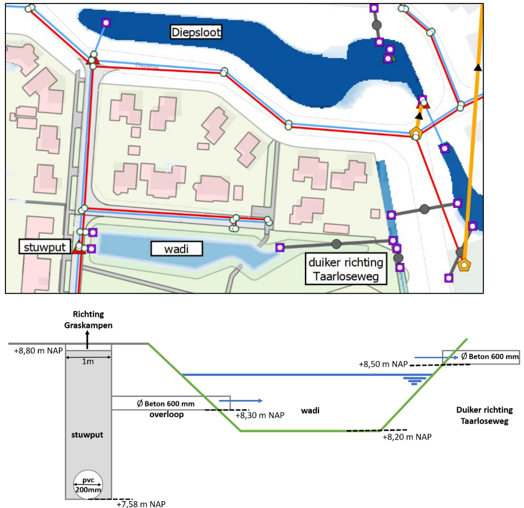
Figuur 3-4: Principe van de stuwput en afwatering wadi. Bij lichte buien stroomt het regenwater af via de doorlaat van rond 200 richting de Graskampen en komt in de vijver bij de Diepsloot terecht. Bij hevige buien voert het regenwater via een rond 600 leiding ook af naar de wadi. Bij het waterniveau van 8,50+ m NAP in de wadi, voert het water via de duiker af richting de sloot aan de Taarloseweg.
