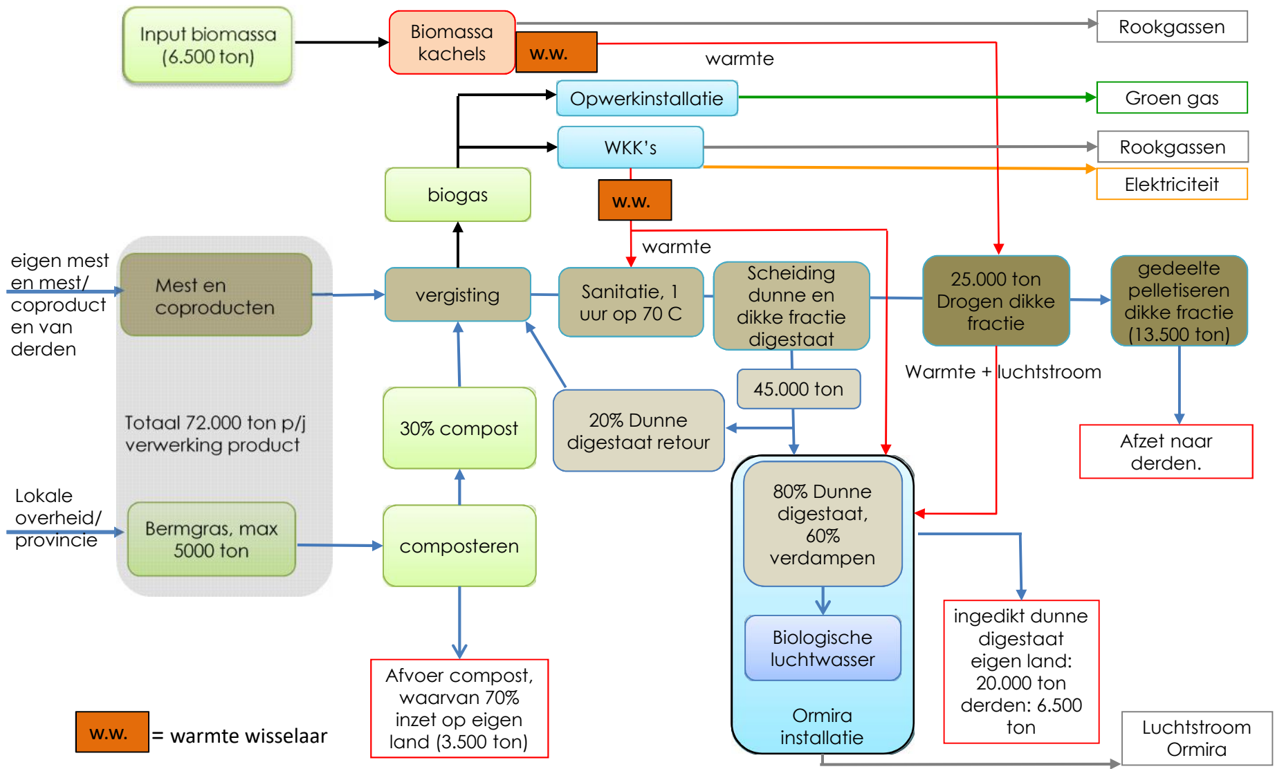
Bijlage proces flow diagramm Mts Hartlief Lammers
