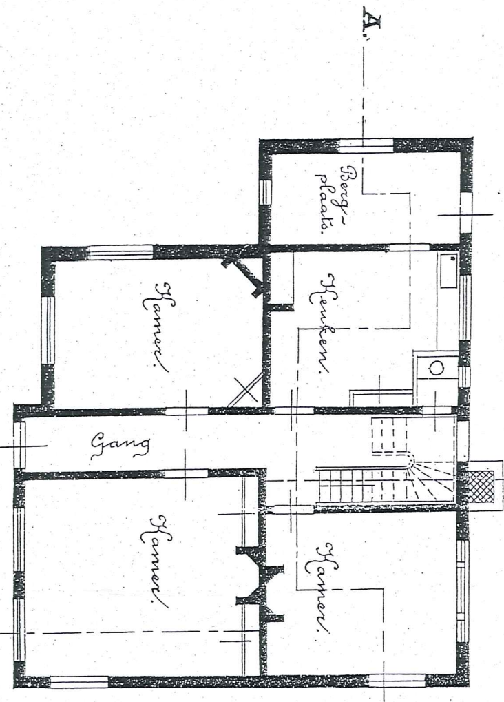
Begane Grond.
