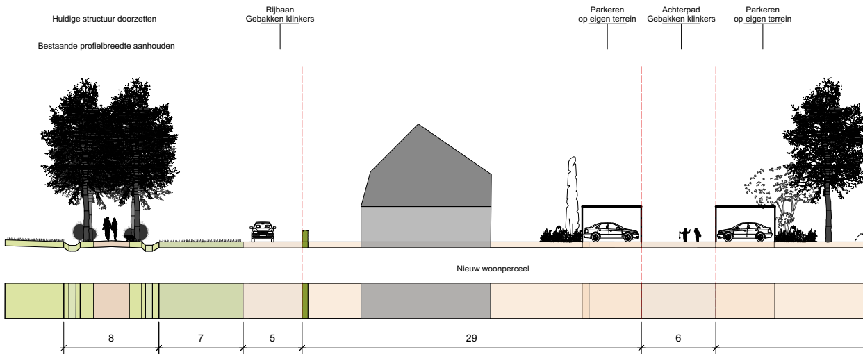
Doorsnede CC
