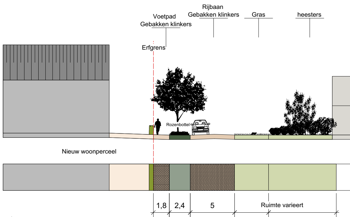
Doorsnede
