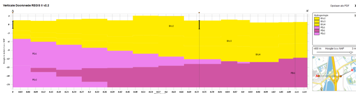
Afbeelding 4.5 Doorsnede van de bodemopbouw uit REGIS II op de locatie van het plangebied
