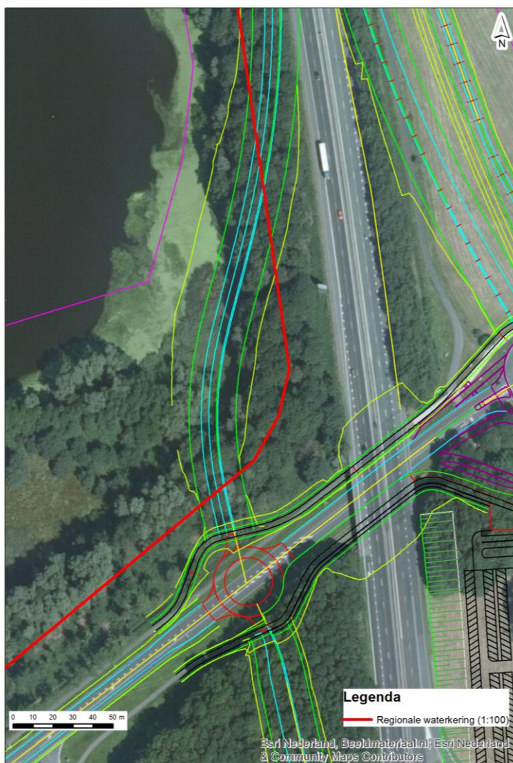
Afbeelding 4.1 Een deel van het ontwerp valt binnen de leggerzone van een regionale waterkering
