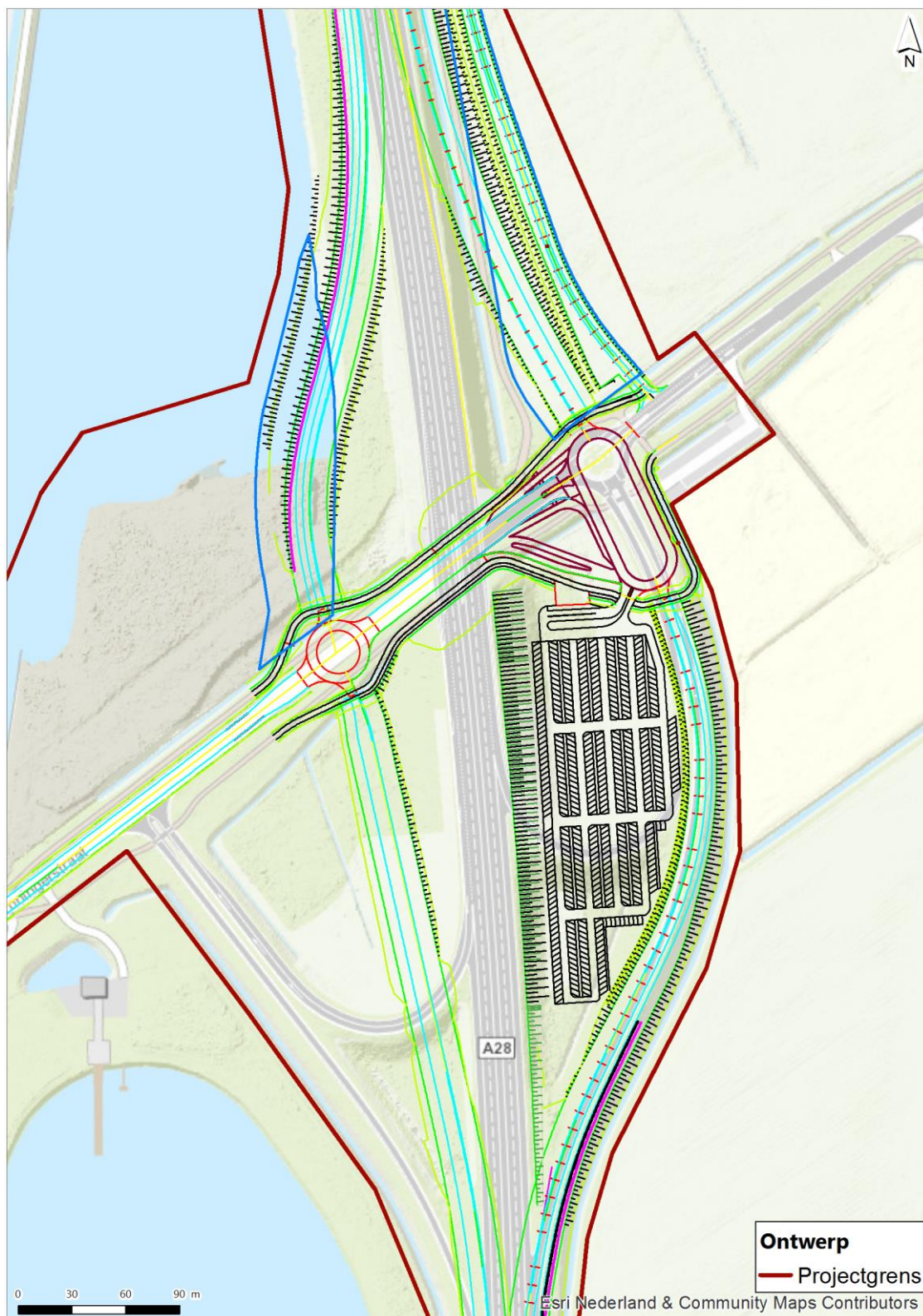
Afbeelding 2.3 Uitsnede uit het concept-ontwerp Transferium De Punt
